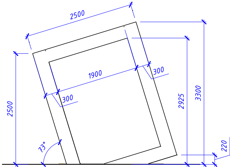
Малая архитектурная форма "Рама-150" М 1:50 (2 шт.)
