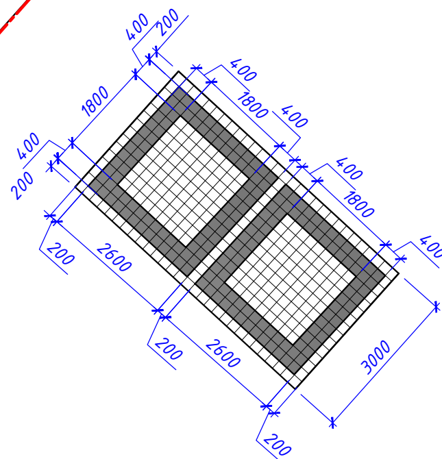
Фрагмент мощения М 1:100
